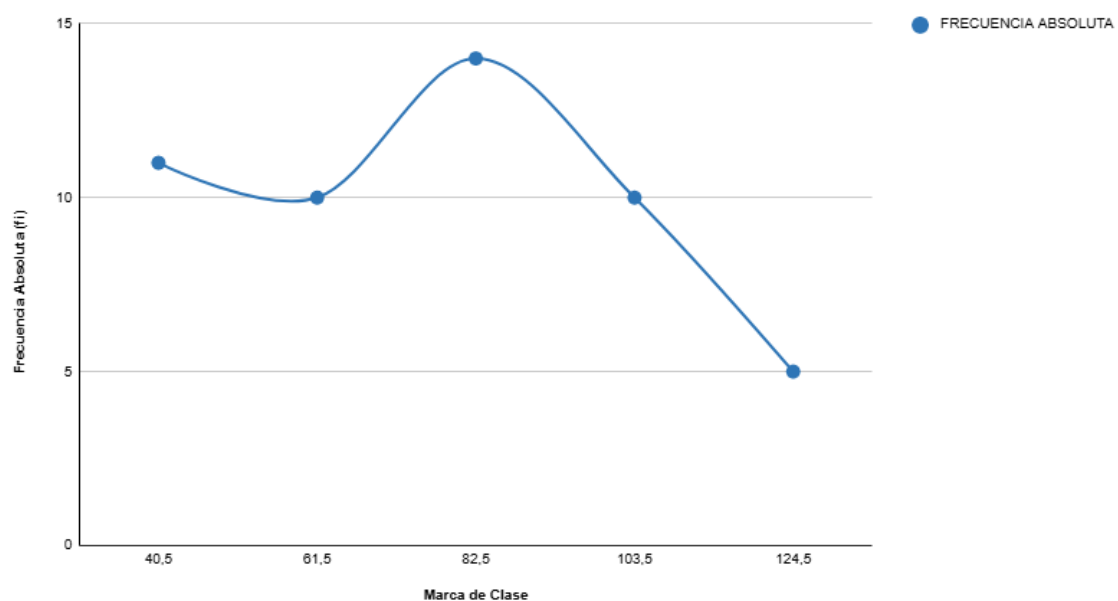
Figura 2. Polígono de Frecuencias – Apps Descargadas
