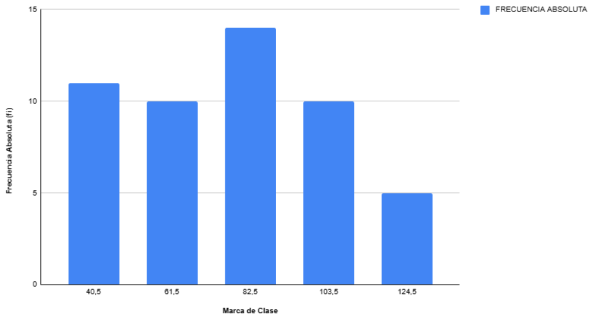
Figura 1. Histograma de Frecuencias – Apps Descargadas
